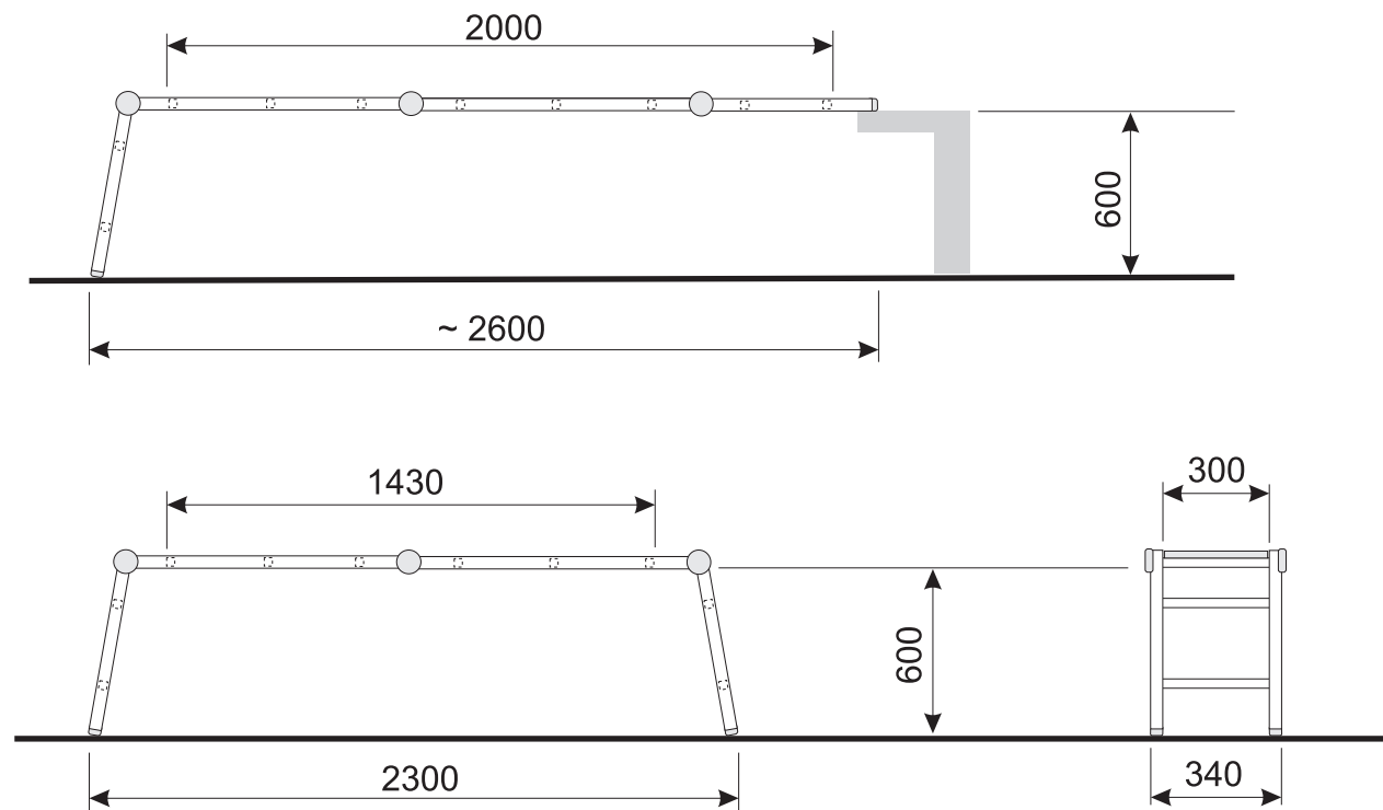
Schemat ustawienia podestu
